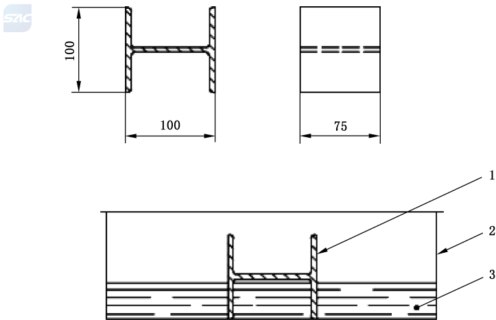
图 F.1 铸件火方盘模型
