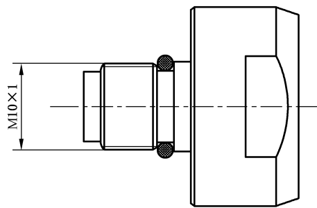
图 D.1 指示器结构型式外形示意图
