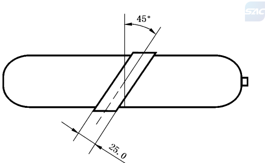
图 B.2 环焊缝瓶体压扁示意图
