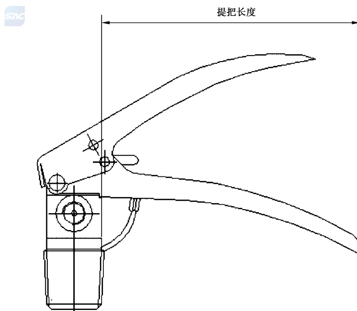
图 C.2 二氧化碳灭火器阀门提把长度示意图
